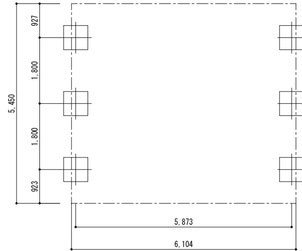
■ 基礎配置図
